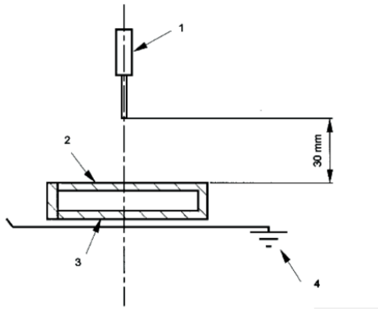
图7 用接地探针通过 0.1 \mu\text{F} 电容给容器放电
