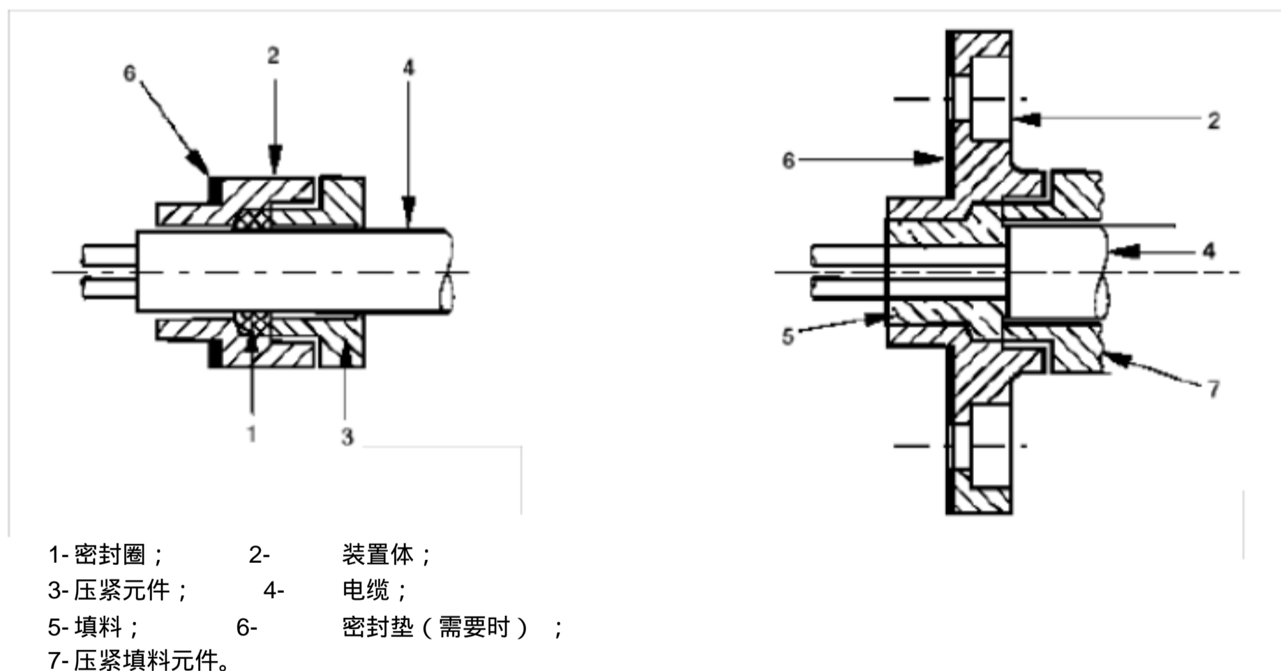
图 A.1 电缆引入装置结构示意图
