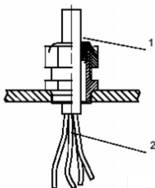
图 3a 电缆引入装置
