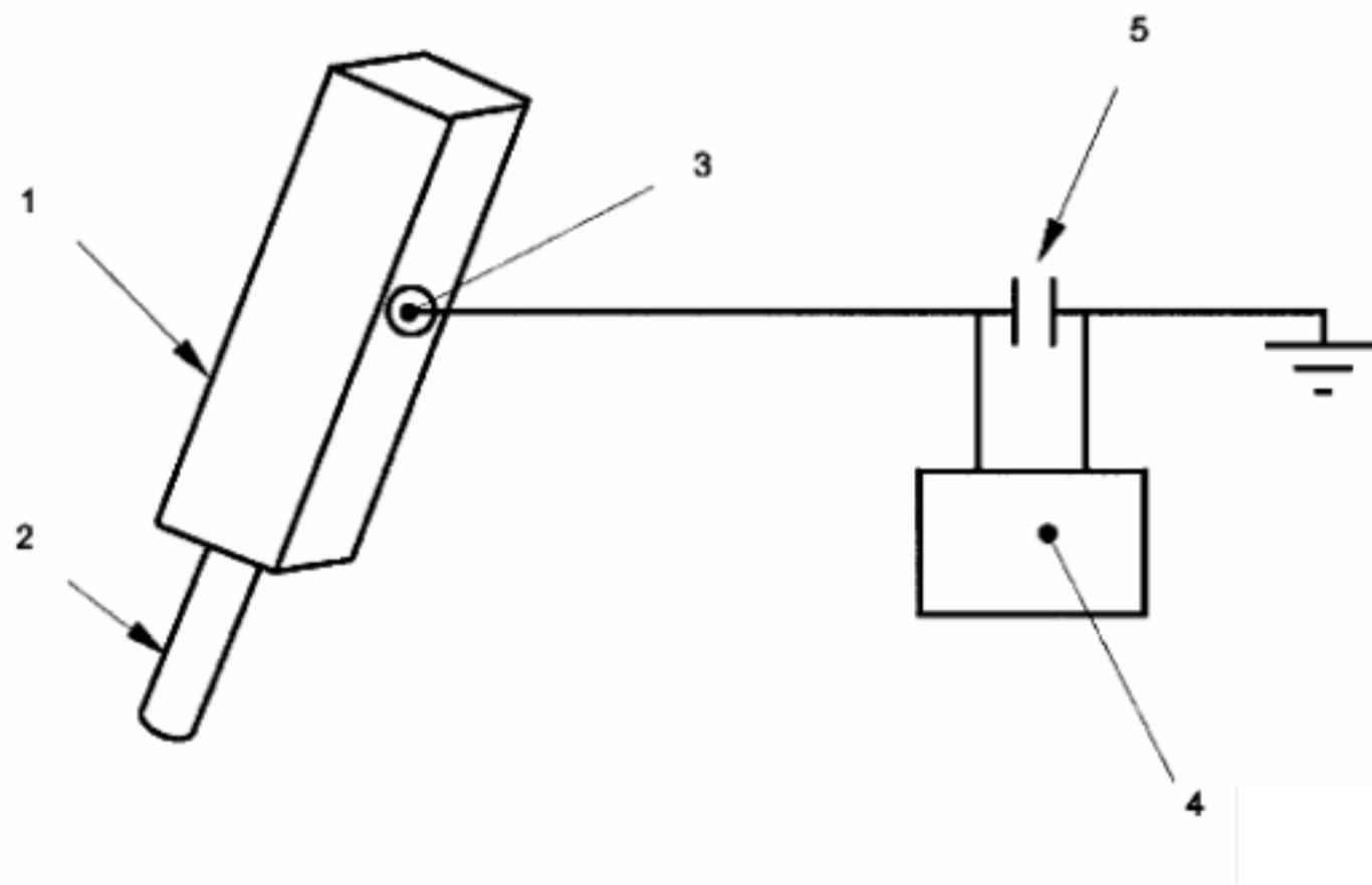
图6 用纯尼龙布或棉布摩擦
